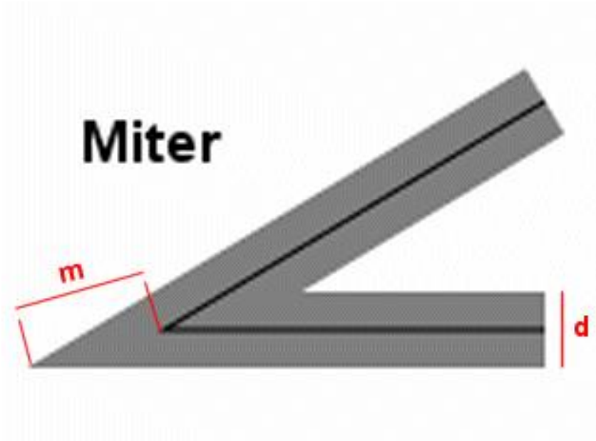
Fig. 7: Miter linejoin
